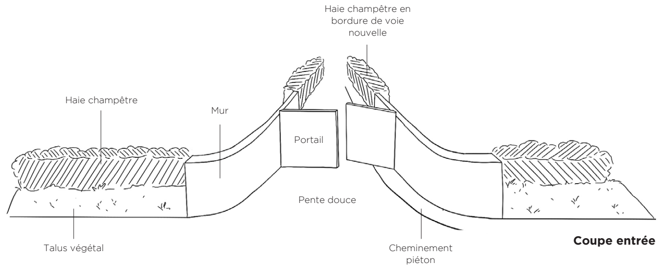
Coupe d'un principe de terrain
